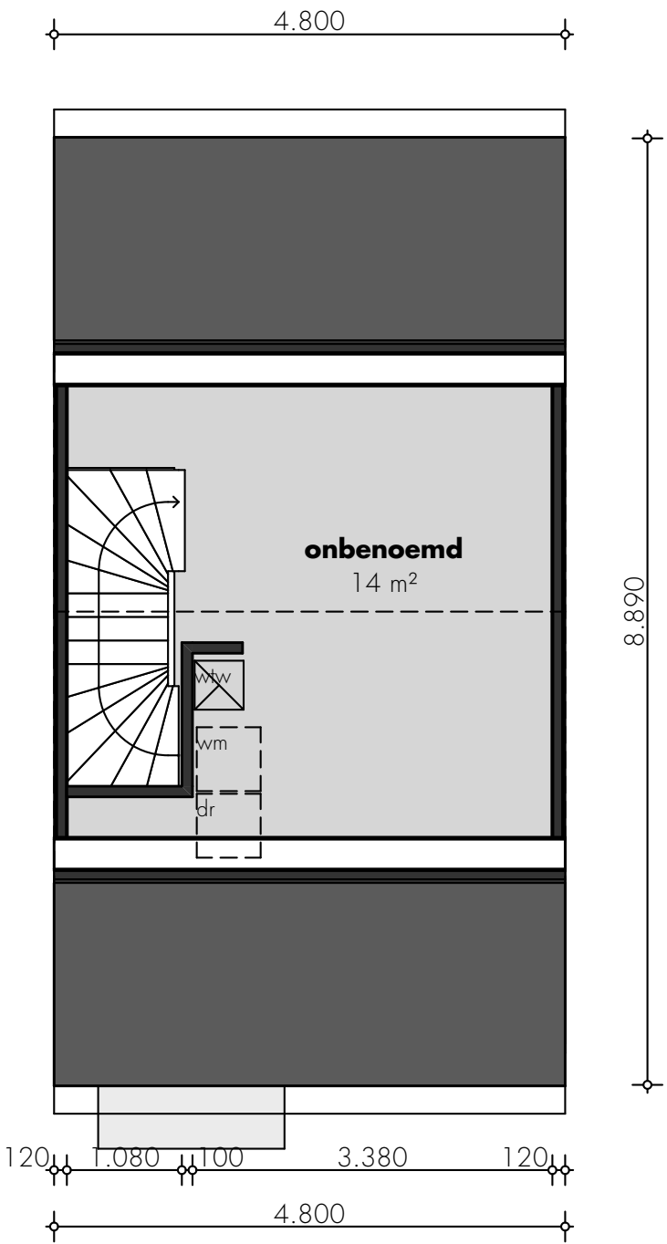
tweede verdieping
