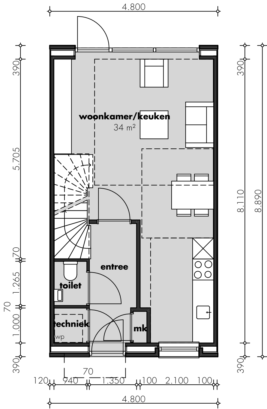
begane grond
